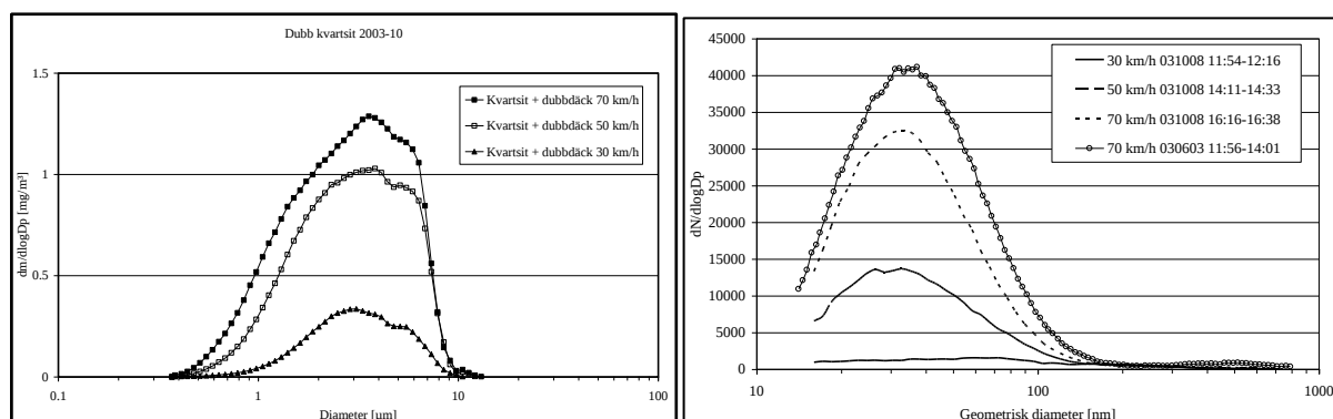
Figur 2. Partikelstorleksfördelning för partiklar mellan 0,523 - 18,47 \mu\text{m} (till vänster) och för partiklar mellan 16 - 723 nm (till höger) vid olika hastigheter i provvägsmaskinen. Kombinationen är ABS med kvartsit och dubbdäck utom den översta kurvan i det högra diagrammet som är ABT med granit och dubbdäck.
