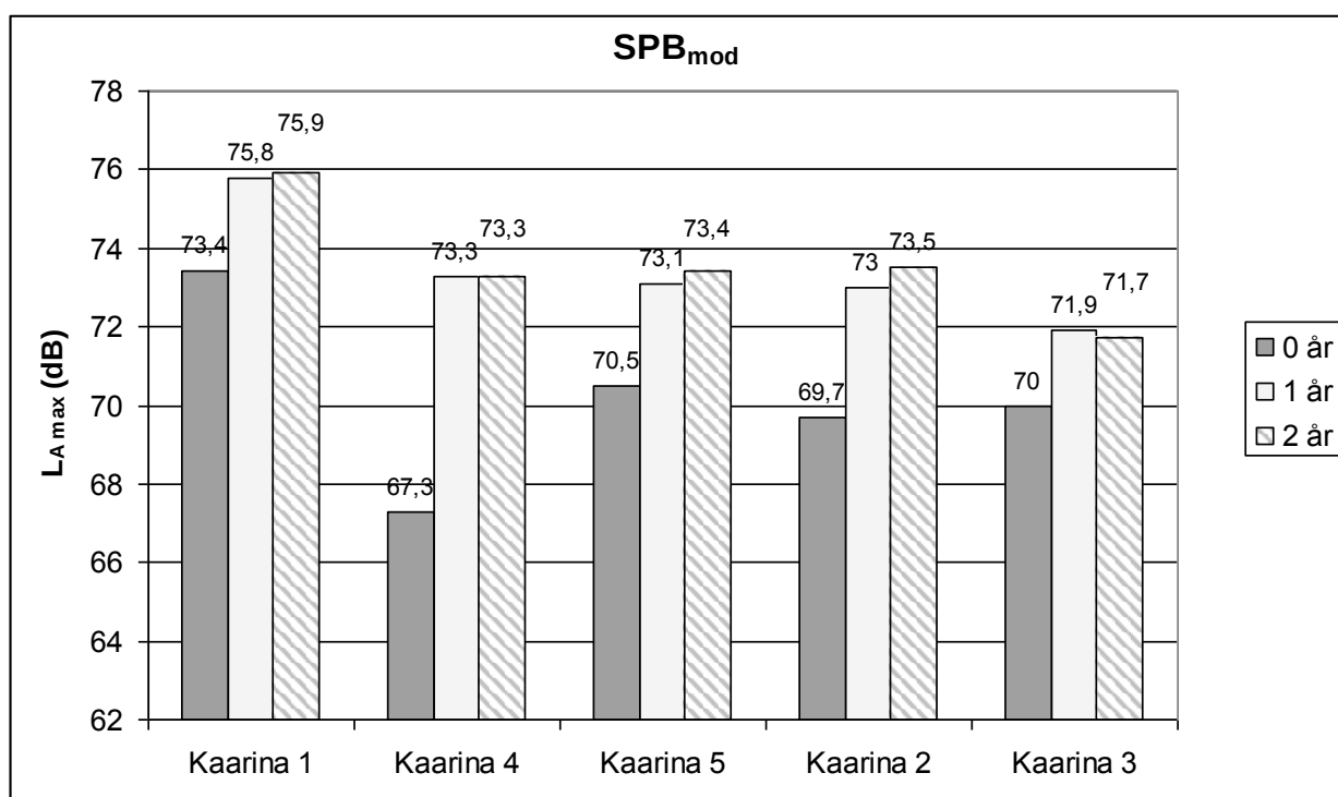
Bild 2: SPB_{mod} - resultat efter ett och två år (Kaarina- testvägen).
