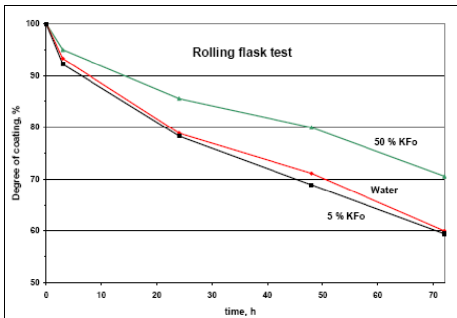
Bild 2: Resultat från rullflask -försök. Det viktigaste resultat är att formiatet har ingen effekt på vidhäftningen mellan stenmaterial och bitumen, när exponering sker i rumtemperatur.
