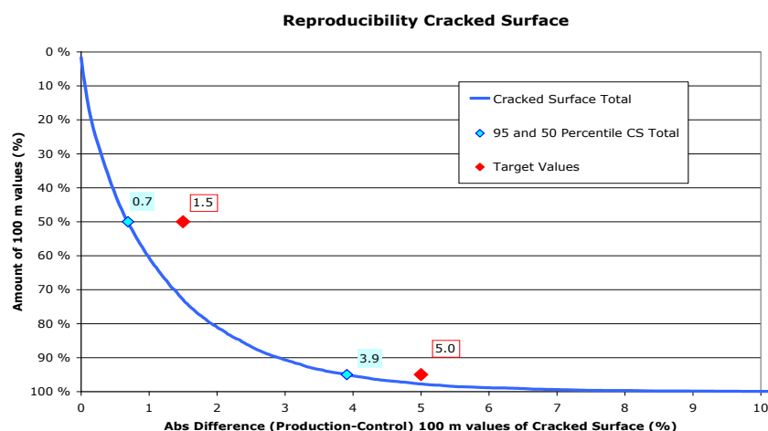
Figur 5. Repetitionsmätningars (produktion- och kontrollmätningar) relativa skillnader och kvalitetskrav för mätningar.
