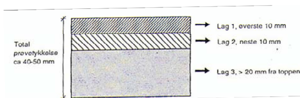
FIGUR 12 Kapping av prøver for bindemiddelgjenvinning
