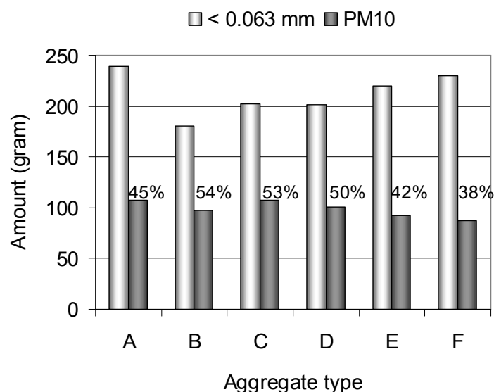
Figur 4. Mengde finstoff < 0.063 mm og andel PM10 generert fra forskjellige bergartstyper (gram) med kulemølle
