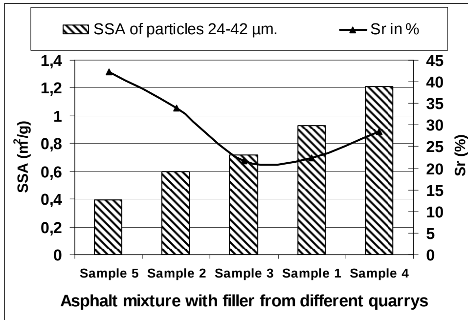
Figur 2 Specifik ytareta (24–42 µm) och styvhetsmodul (Sr) efter 35 frys –tö cyklingar(omarbetad efter Said m.fl. 2007).
