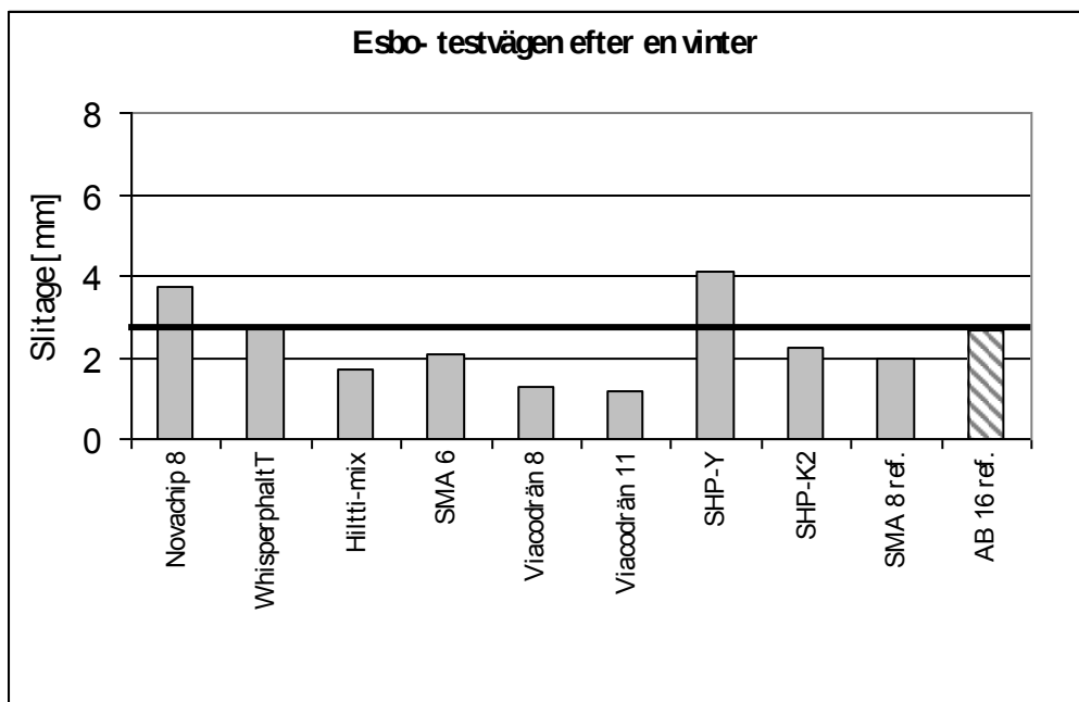
Bild 3: Slitage av tysta och referensbeläggningsarna.
