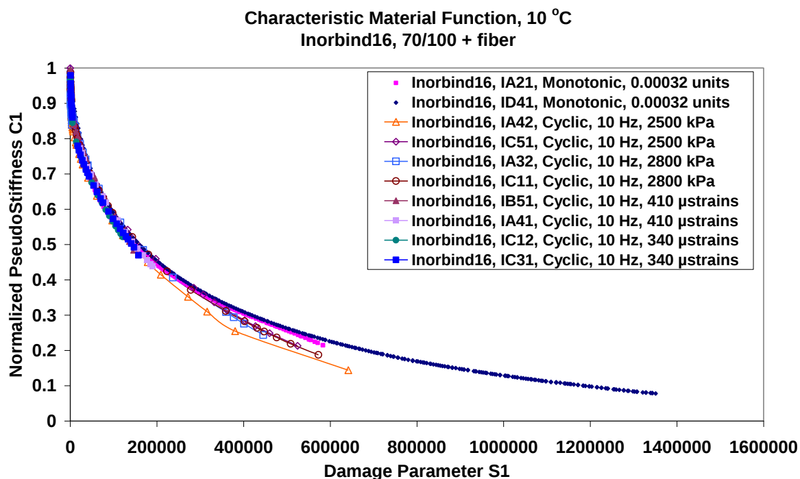
Figur 1 C_1 vs. S_1 , Inorbind16™, monotoniska and cykliska tester (10 Hz), 10 °C, \alpha=(1+1/m) .
